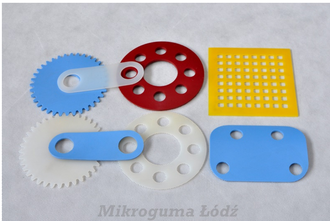
uszczelki wycinane
